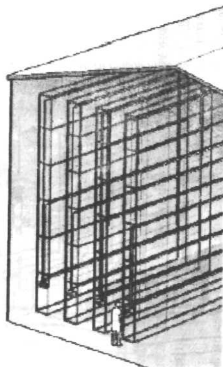
Рис. 4. Горизонтальный отбор проб в стеллажах
