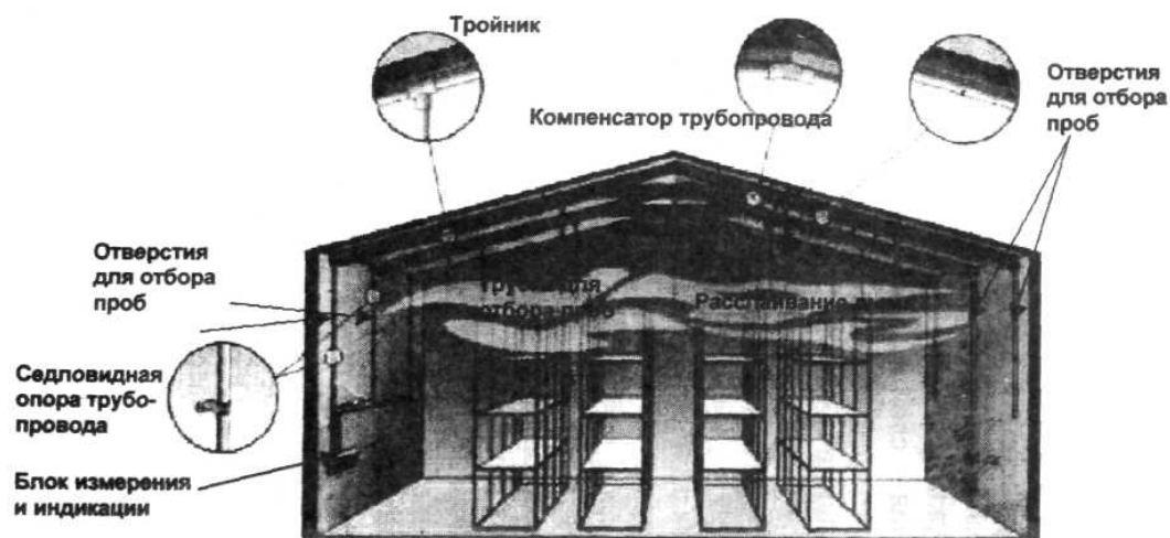
Рис. 3. Конфигурация сети заборных трубопроводов и блоков измерения и индикации аспирационных пожарных извещателей VESDA
