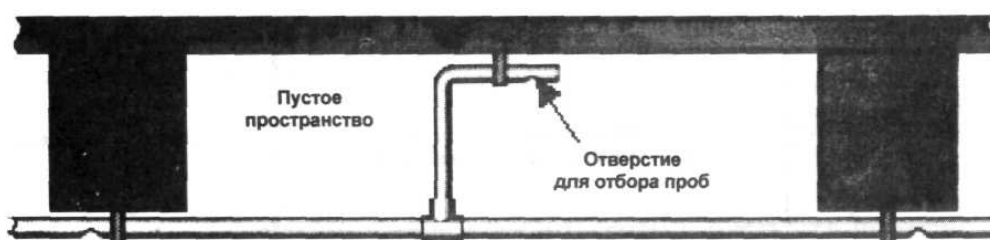
Рис. 8. Заборный трубопровод с использованием капилляров типа "трость"
